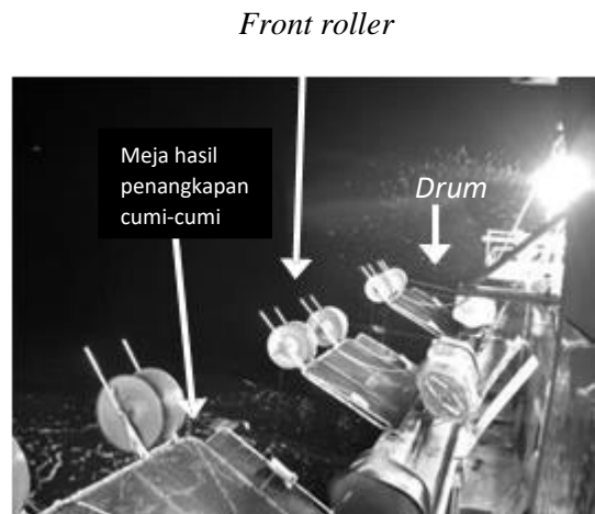
Gambar 8: Mesin pancing cumi-cumi otomatis sedang beroperasi
