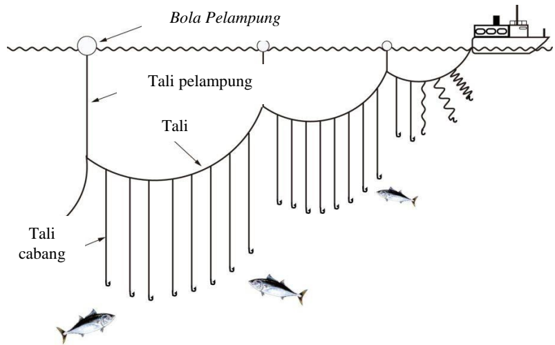
Gambar 11: Skema Penangkapan Rawai Ikan Tuna
