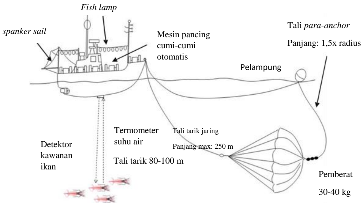
Gambar 6: Kapal penangkap cumi-cumi
